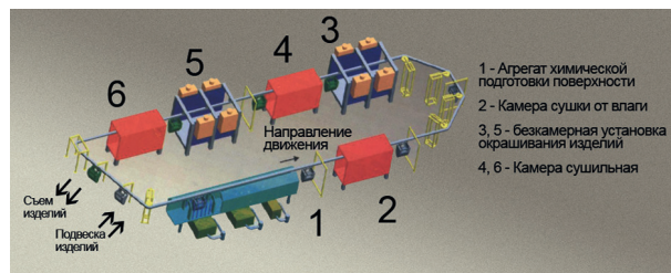
Автоматизированная покрасочная линия
